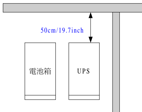
圖 4-1 通風 (上視圖)
