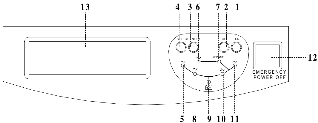
圖 1-1 前控制面板
