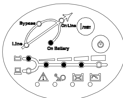
4-1 電池模式
