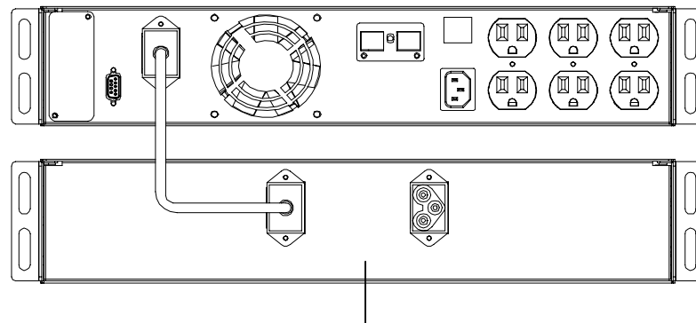
外接電池箱
