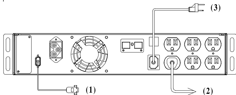
3-4 UPS 連接
