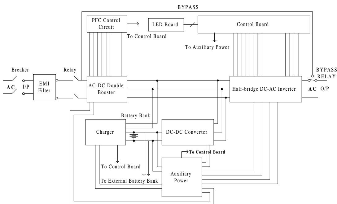
2.1 UPS 系統方塊圖
