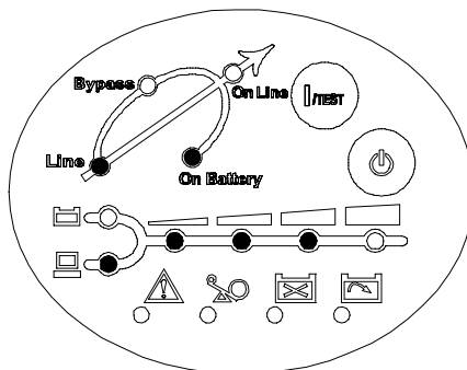
4-3 UPS 自我測試
