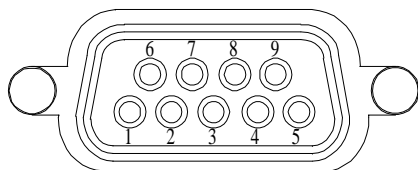
8-1 腳位配置
